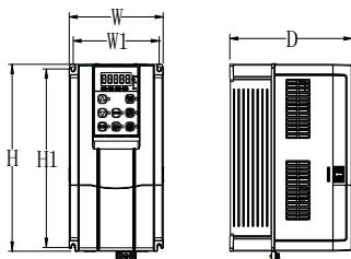
图 2-4. TA300(S)系列 11KW 以下塑胶外形尺寸及安装尺寸示意图 (TA300N 22KW 以下为塑壳机箱)
