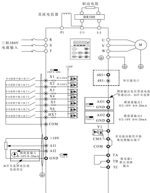
图 3-4.93Kw (4T:380V 93 Kw) 及以上三相变频器
