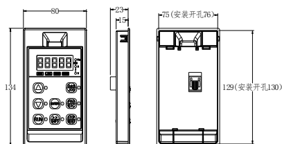
图 2-8.3 大号外引键盘带托盘安装尺寸图 (TA300(S)系列 4T:380V 55kW 以上标配大号外引键盘, TA300N 系列 4T:380V 15~22Kw, 55Kw 以上标配大号外引键盘)
