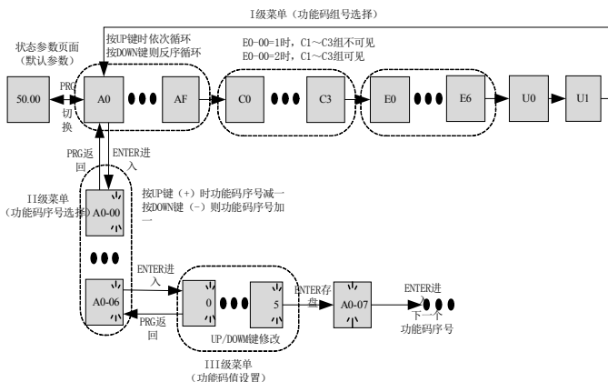
图 4-2. 三级菜单操作流程图
