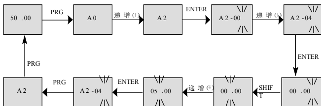
图 4-3. 参数设定操作流程图
