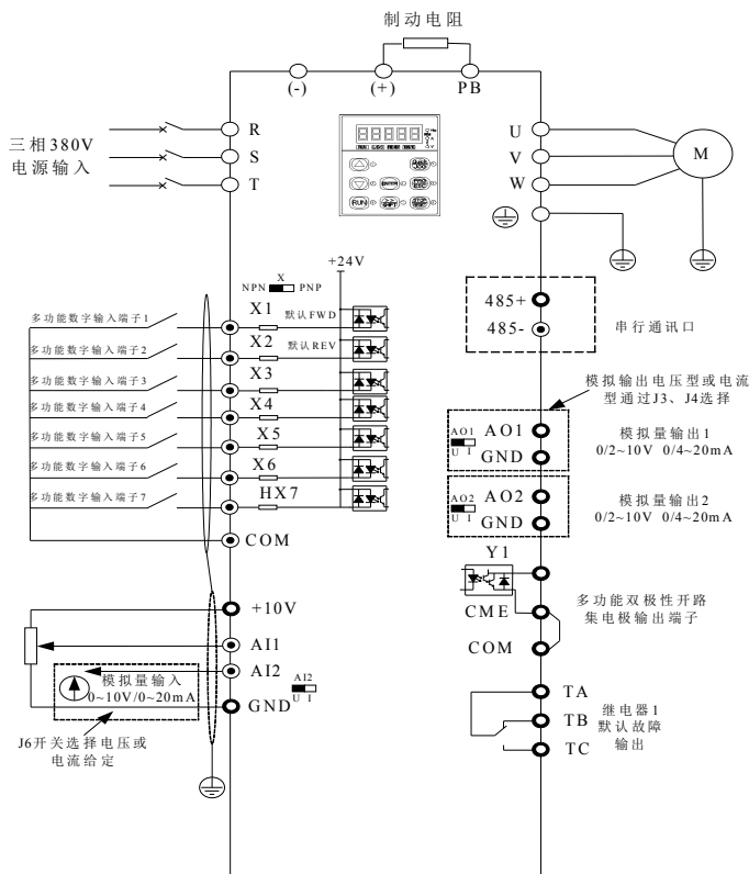
图 3-2. TA300(S)系列 4.0~ 30kW(4T:380V 4.0 ~ 30kW), TA300N 系列 7.5~ 30kW (4T:380V 7.5 ~ 30kW) 三相变频器接线图
