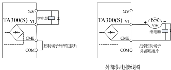
图 3-12. 数字输出端子 Y1 接线示意
