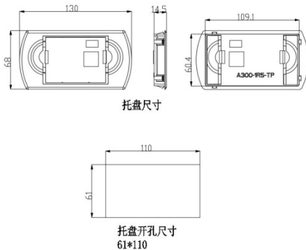
图 2-8.1 小号外引键盘带托盘安装尺寸图 (TA300(S)系列 4T:380V 2.2kW 以下标配小号外引键盘, TA300N 系列 4T:380V 5.5kW 以下标配小号外引键盘)
