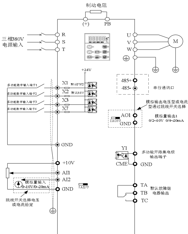
图 3-1. TA300(S)系列 2.2kW (4T:380V 2.2 kW) 及单相 220V 2.2kW 以下 220V 接 R T 或 L N, TA300N 系列 5.5kW (4T:380V 5.5 kW) 以下三相变频器接线图
