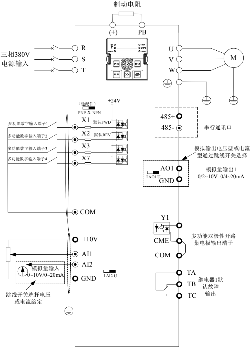
图3-1. 三相380V 2.2kW (4T:380V) 及单相220V (2S) 1.5kW(输入接L N或R T)以下变频器接线图 备注：数字输入端子X跳线开关出厂默认NPN模式（即X短接COM有效），PNP模式为选配功能，三相380V 2.2 kW及单相220V 1.5 kW以下如需选配PNP模式，订货时请说明。AI2, AO1跳线开关出厂默认电压模式。
