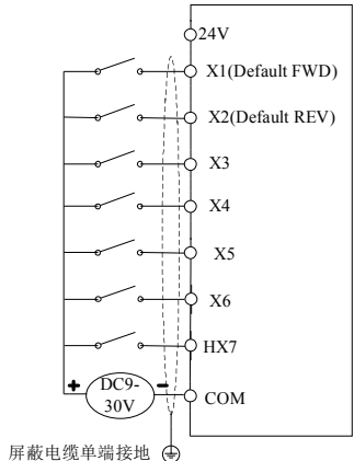
图 3-11. 四种不同模式下数字输入端子接线图
